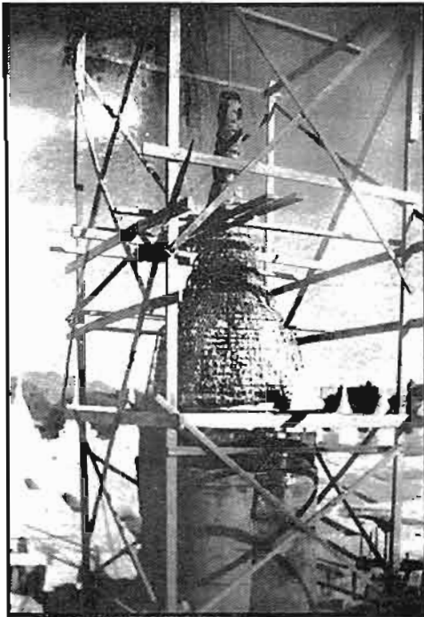
အမိုးပြားပေါ်တွင် ခေါင်ပွစေတီတည်ဆောက်
