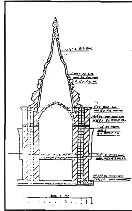
သံကွန်ကရစ် စေတီ စနစ်ပုံ
